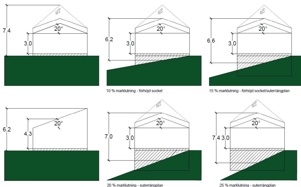
Illustrationer för hur byggnader kan utformas utifrån plankartans bestämmelser.
